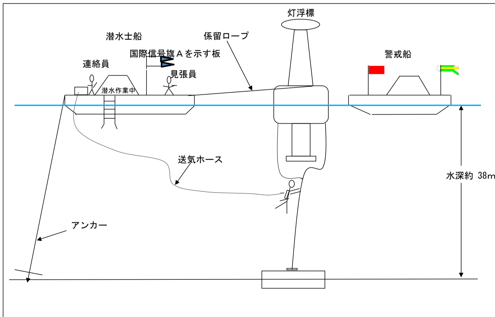
図-2. 施工概要図
