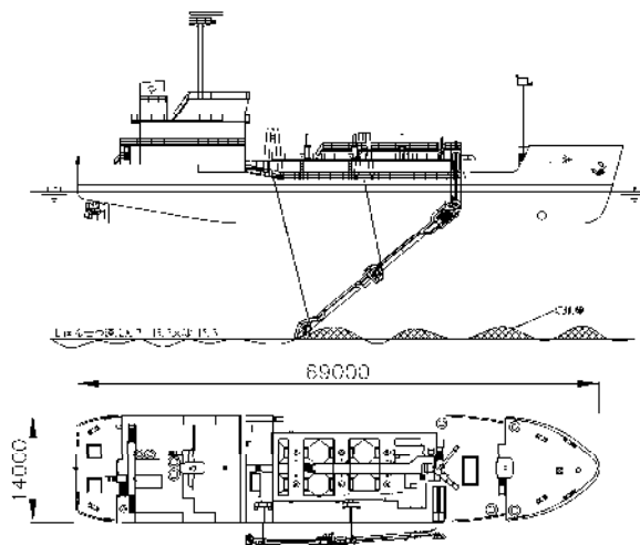
浚渫船「海竜」しゅんせつ作業状況図
