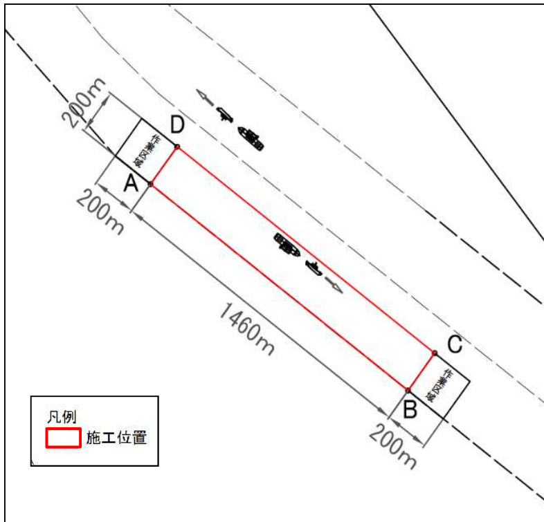
浚渫船「海竜」しゅんせつ作業状況図
